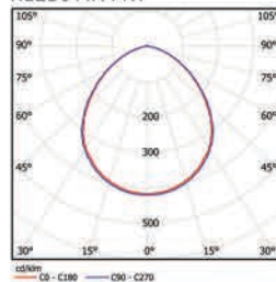
NLED944A 14W
