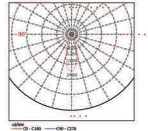
TLED332D 20W
