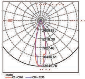
TLED319N 50W 24°
