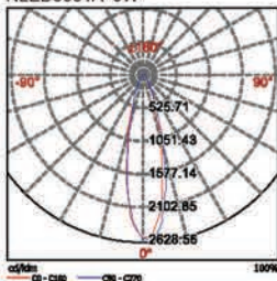
NLED5851A 9W
