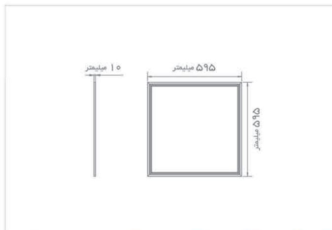
فریم جهت نصب روکار
