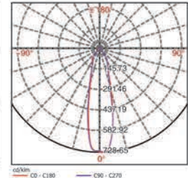
NLED1102D 12W
