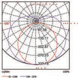
T8E 18W
